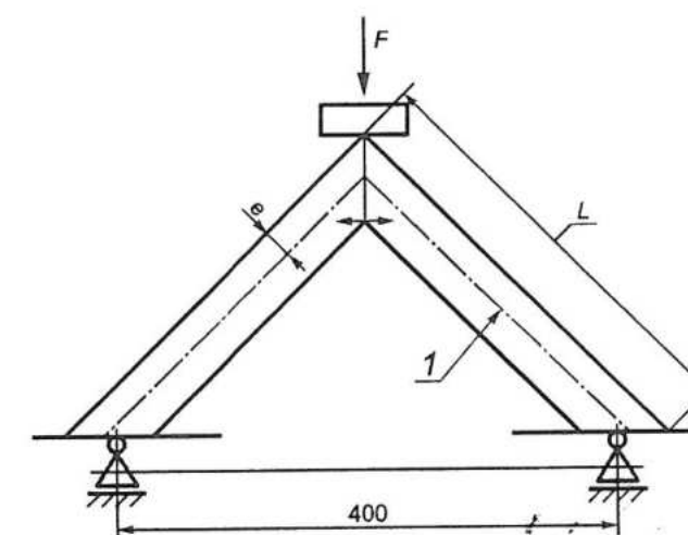
1 — нейтральная ось профиля длиной 283 мм; F — вертикальная сжимающая нагрузка на угловое соединение; L — длина стороны угла по наружной поверхности; e — расстояние от оси до кромки профиля
