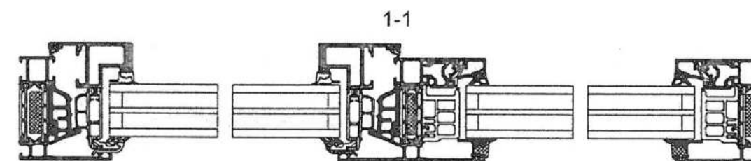
Рисунок 10 — Пример конструктивного решения алюминиевого оконного блока с комбинированным открыванием: глухая (неоткрывающаяся) и поворотно-откидная створка, открывающаяся внутрь помещения
