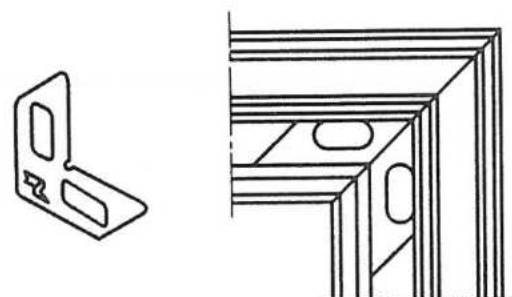
а) Крепежный уголок
