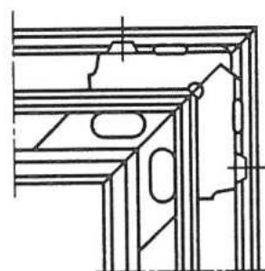
в) Соединение крепежным уголком с дополнительной фиксацией винтами
