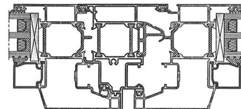
Рисунок 6 — Пример конструктивного решения штапикового притвора
