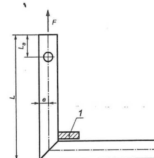
1 — устройство для фиксации профиля; F — вертикальная нагрузка растяжения на угловое соединение; L — длина стороны угла по наружной поверхности равная 300 мм; L a — расстояние от отверстия до торца профиля длиной 100 мм; e — расстояние от оси до кромки профиля
