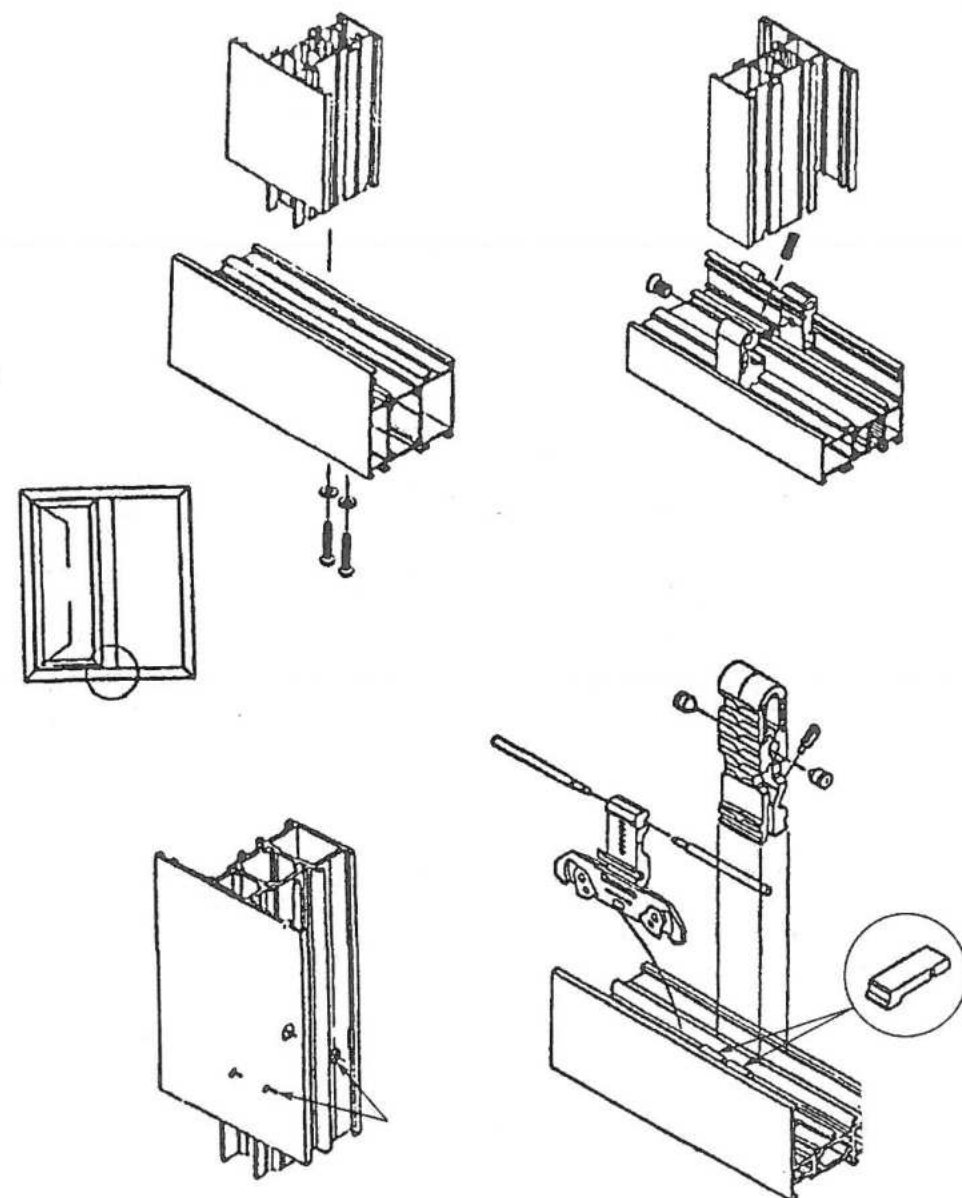
Рисунок А.4 — Примеры конструкций узла крепления импоста
