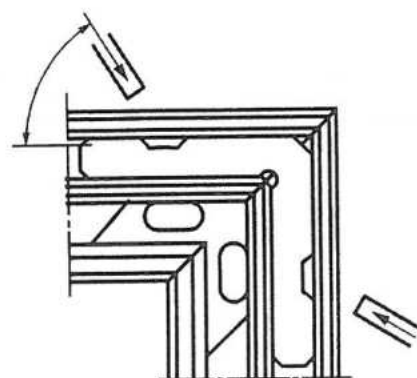
б) Соединение крепежным уголком с обжатием (опрессовкой)
