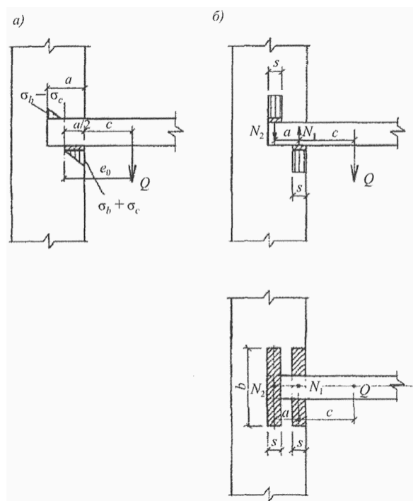
9.4-сүрөт – Консоль устундарын орнотуунун схемалары
