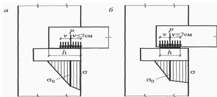
а – бекитүүчү төшөмсүз устунду колдоо; б – устунду төшөм менен колдоо
