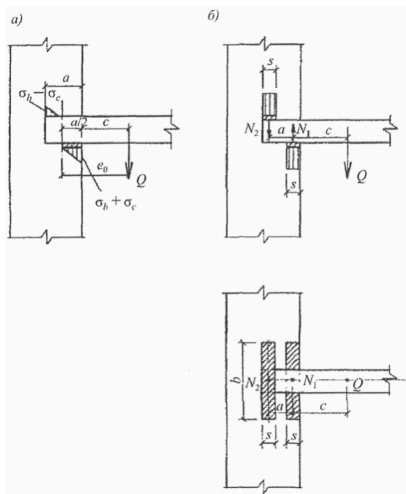
Рисунок 9.4 – Расчетные схемы заделки консольных балок
