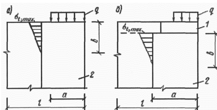
a – при отсутствии распределительной плиты; b – при установке распределительной плиты; 1 – распределительная плита; 2 – кладка
