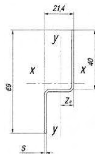
Рис. Г.9 – Профиль Z-образный 70
