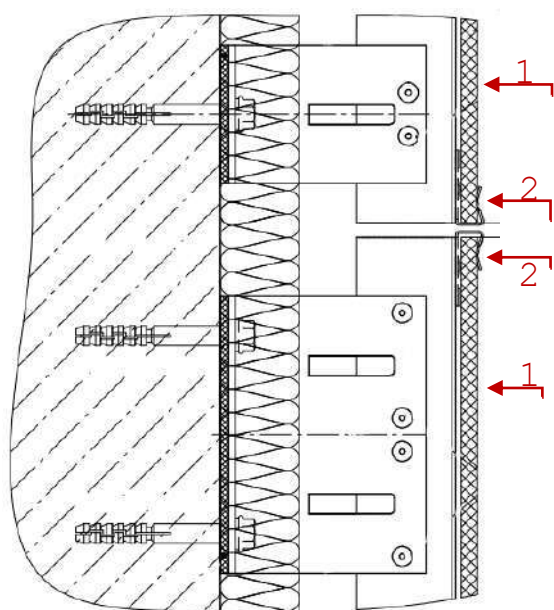
Верное крепление
