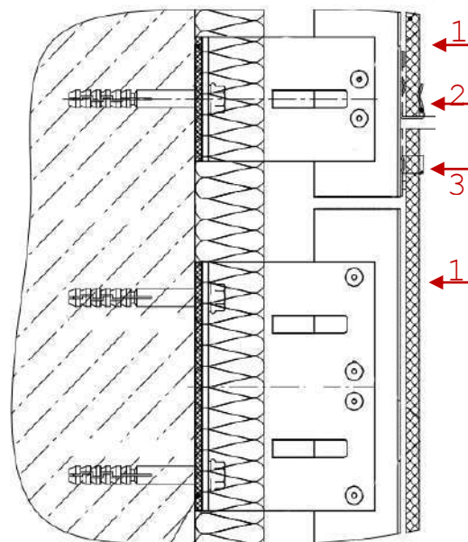
Верное крепление
