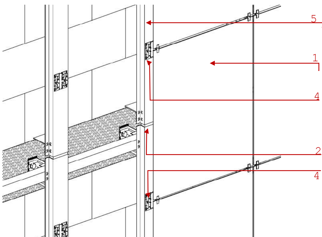
Неверное крепление
