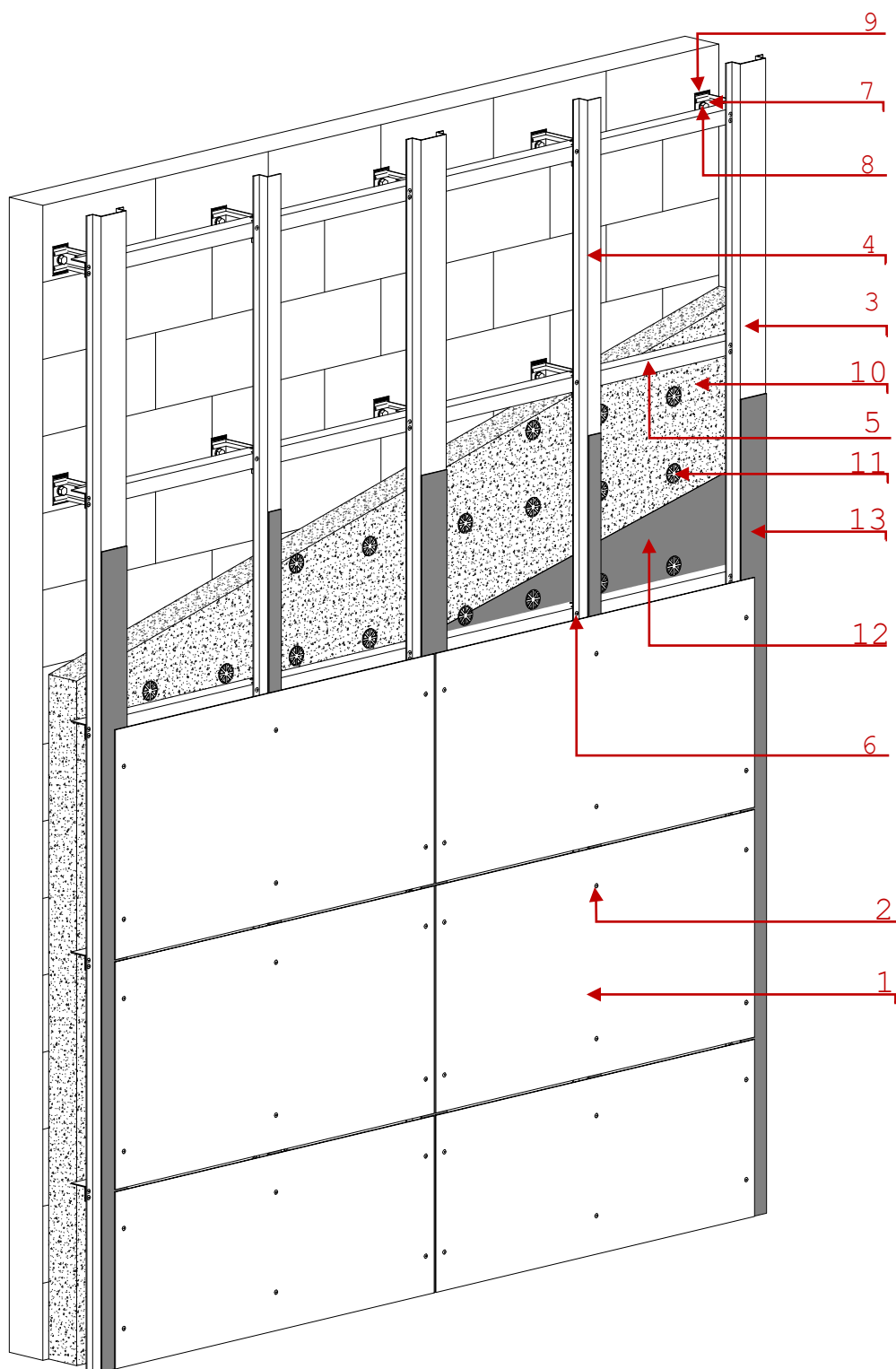
Схема установки облицовочных плит из фиброцементных панелей 600x1200x8 мм на перекрестно-балочную подсистему:
