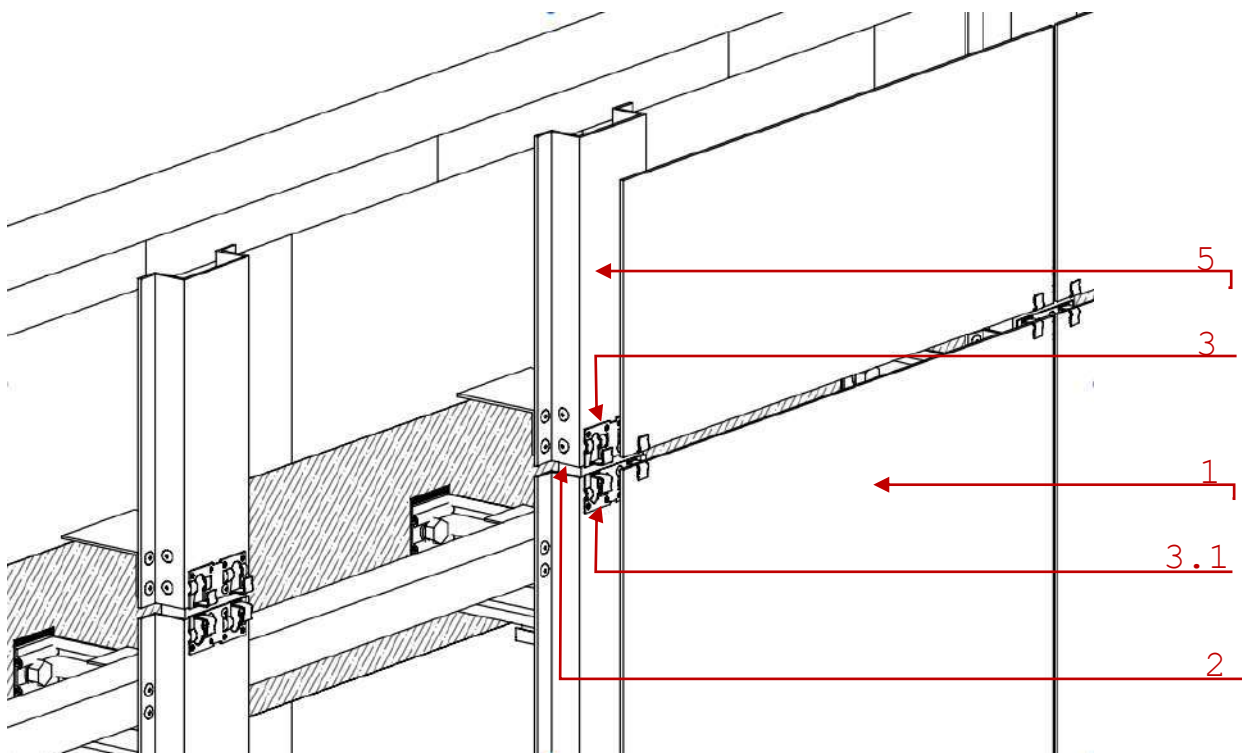
Верное крепление
