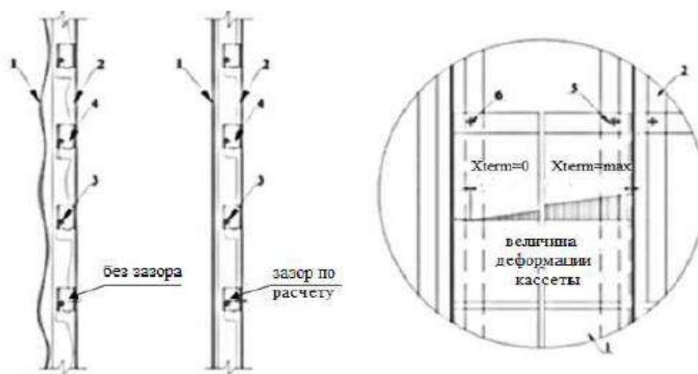
Рисунок 9.4 – Схема закрепления кассеты с учетом компенсации термических деформаций
