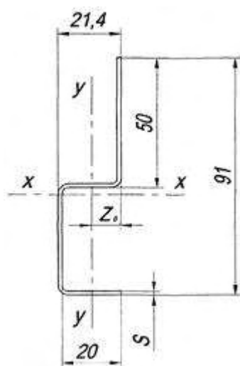
Рис. Г.8 – Профиль Z – образный усиленный
