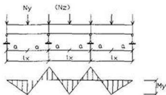
Рисунок Д2 – Расчетные схемы горизонтальной направляющей P z и N z – вертикальные нагрузки (не показаны)
