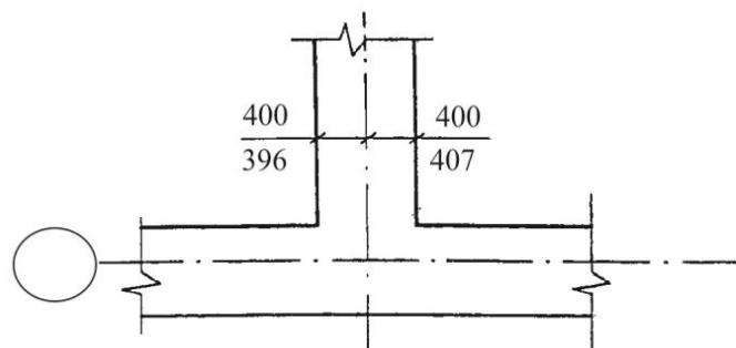
а) От граней монолитного ростверка до разбиваемой в натуре координационной оси
