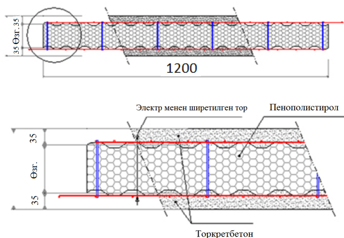
Г.1-сүрөт – Торкретбетондун эки катмары менен бир кабат панель
