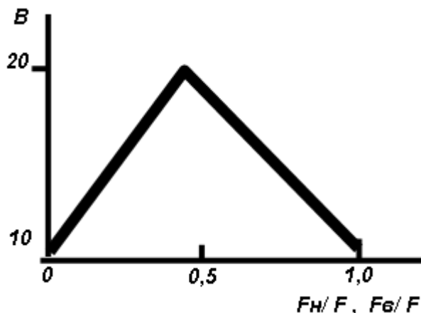
И.1-сүрөтү – k_4 коэффициентти эсептөөдө В коэффициентин аныктоонун графиги
